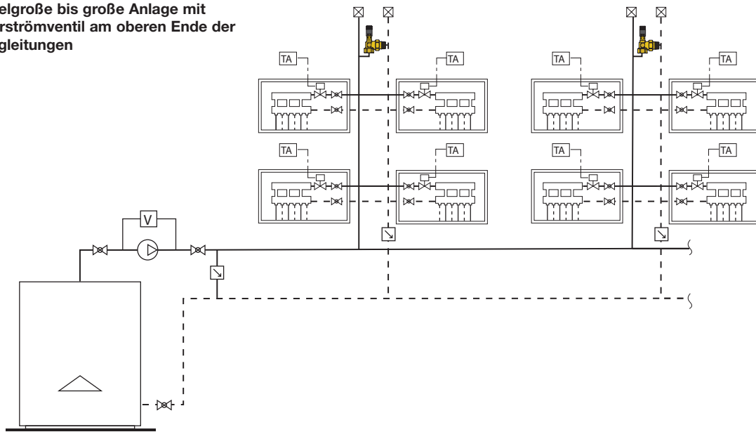
Anlage mit Wärmepumpe, Bypass in Zentrale
